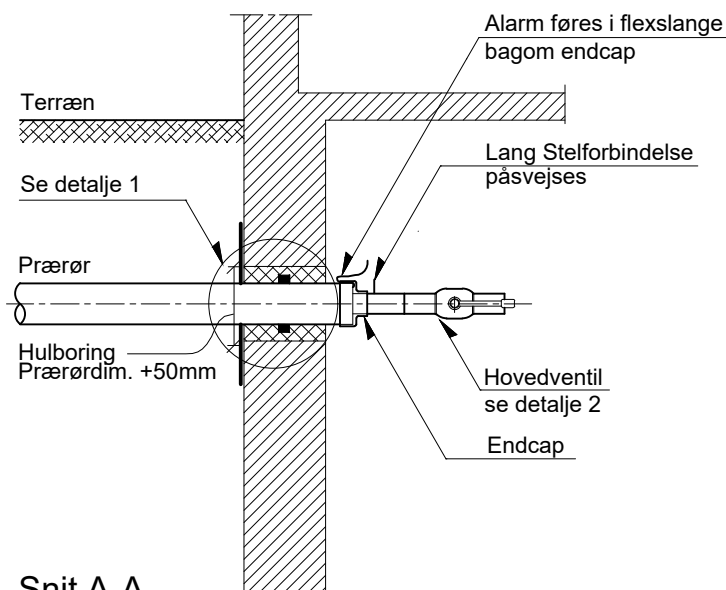
Snit A-A
